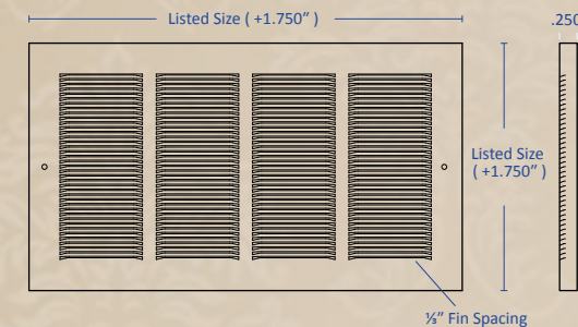
Model 173 • 1/3" Fin Spacing
