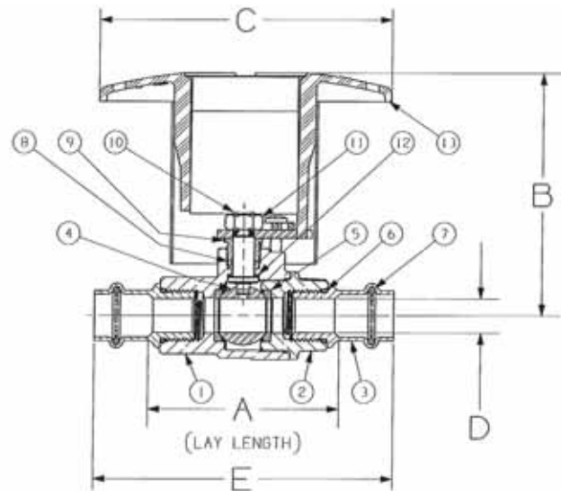
PC585-70-66-NS P x P
