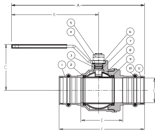
PC-FP-600A-LF
