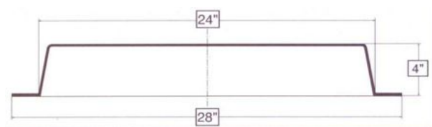
DOME DIMENSIONS
