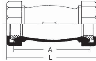
440L Coupling – Long (Galv)
