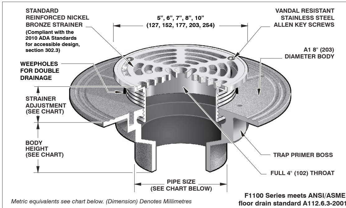
A1 BODY
