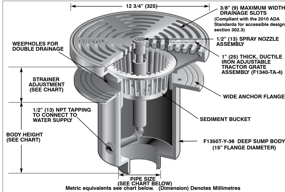
F1350T-Y-36 Body
