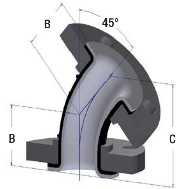
45° Elbow
