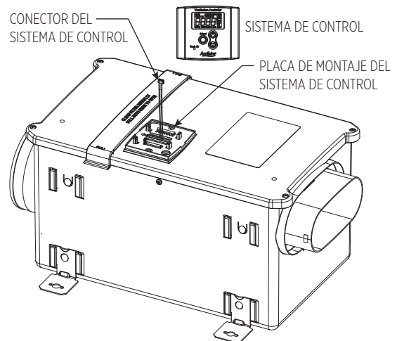
FIGURA 9: RETIRO DEL SISTEMA DE CONTROL DE LA PLACA DE MONTAJE
