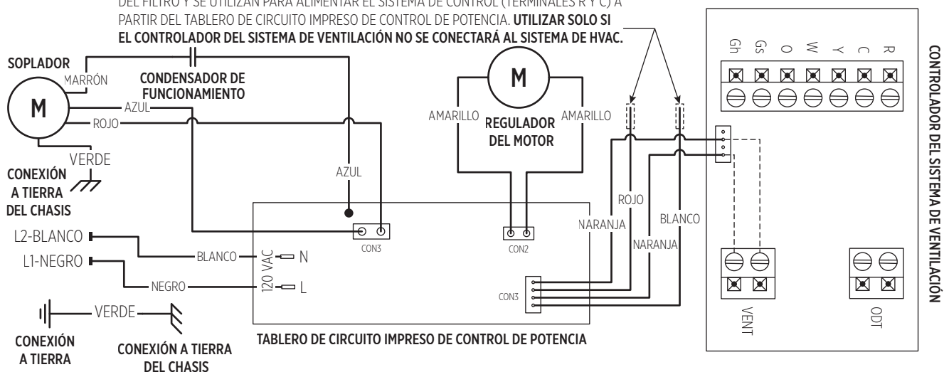
FIGURA 15: ESQUEMA INTERNO DEL MODELO 8145
