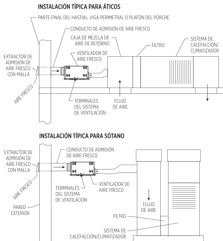
FIGURA 5: INSTALACIÓN DE LOS CONDUCTOS EN SISTEMAS DE HVAC CON FLUJO DE AIRE ASCENDENTE Y HORIZONTAL
