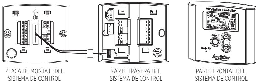
FIGURA 12: CONEXIÓN DEL SISTEMA DE CONTROL AL VENTILADOR
