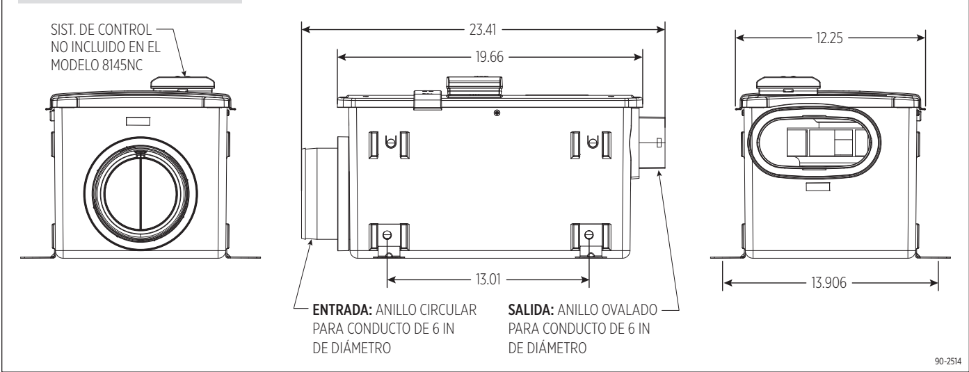
FIGURA 1: DIMENSIONES (PULGADAS)
