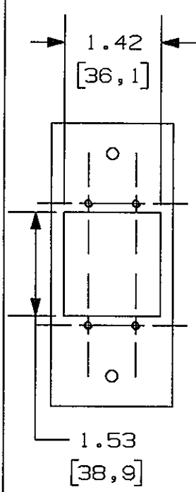
CATALOG NUMBER S1R8CSP1 1-G DUPLEX
