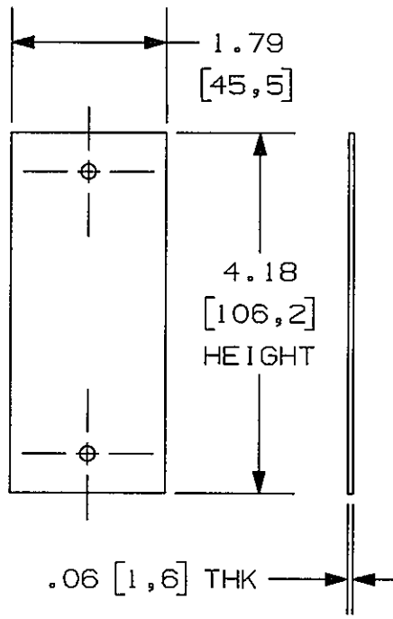
CATALOG NUMBER S1R8CSPB 1-G BLANK PLATE
