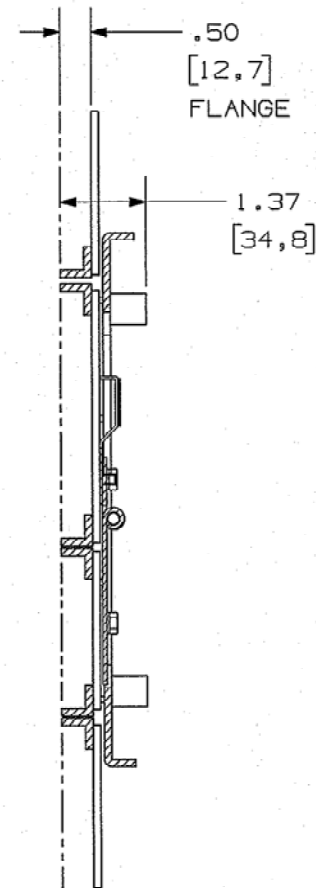
SECTION A-A
