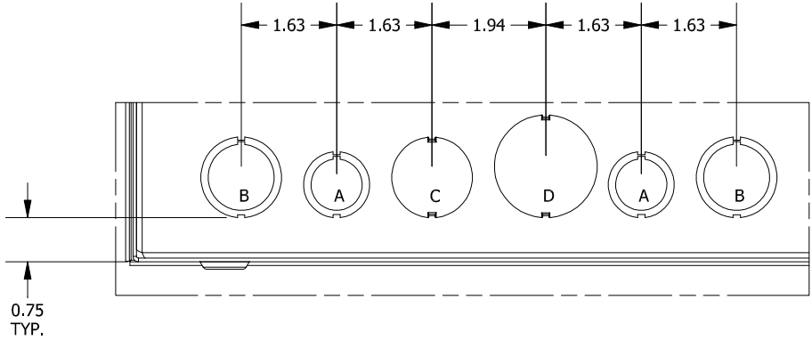
DETAIL B (3 PL.) (K.O. PATTERN)
