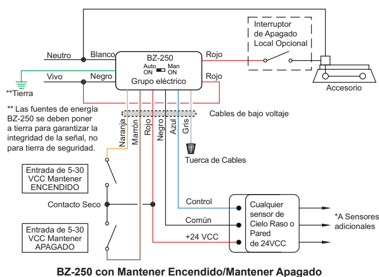
BZ-250 con Mantener Encendido/Mantener Apagado
