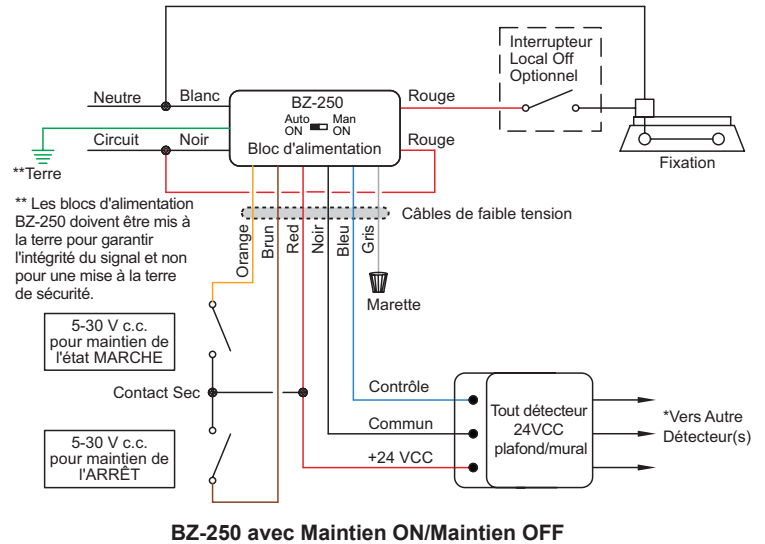
BZ-250 avec Maintien ON/Maintien OFF
