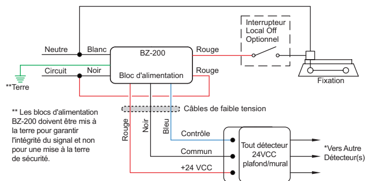
Raccordement pour un BZ-200
