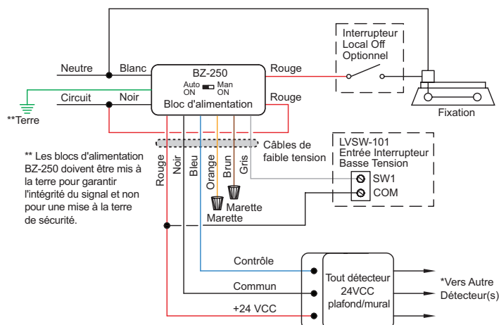
Raccordement pour un BZ-250
