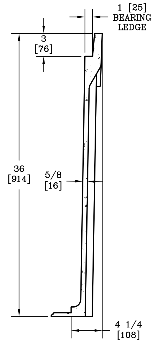
SECTION A-A SCALE: 1 1/2"=1'
