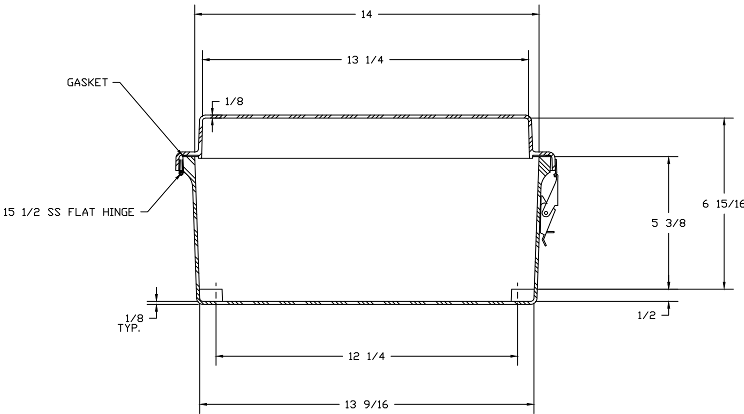
SECTION A-A
