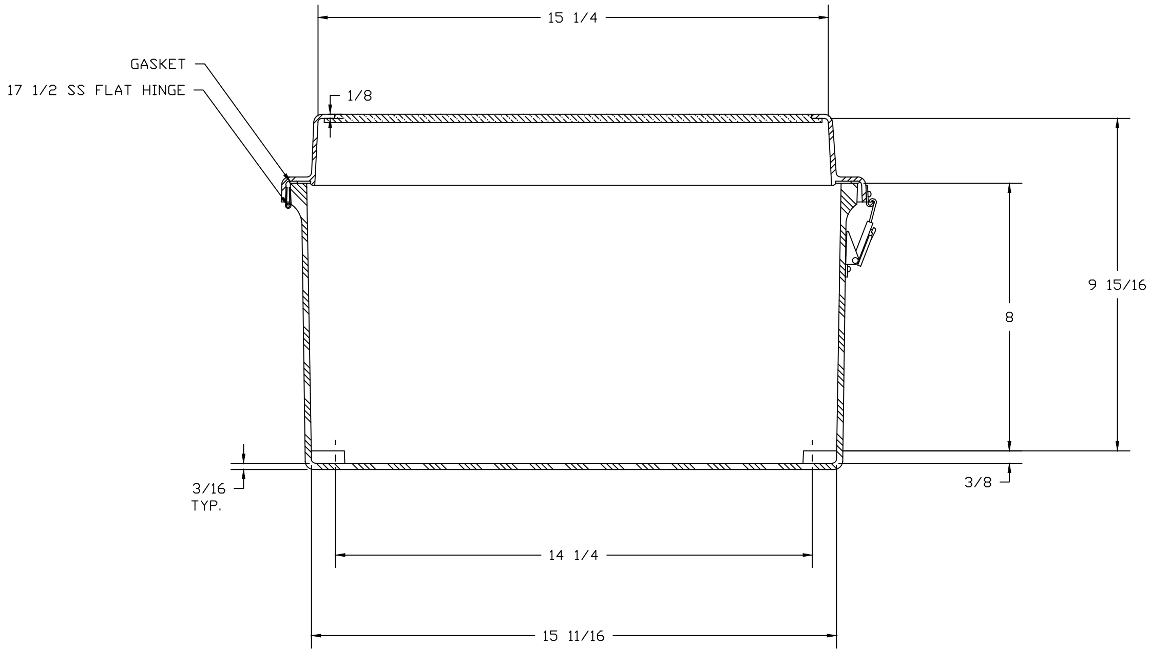
SECTION A-A
