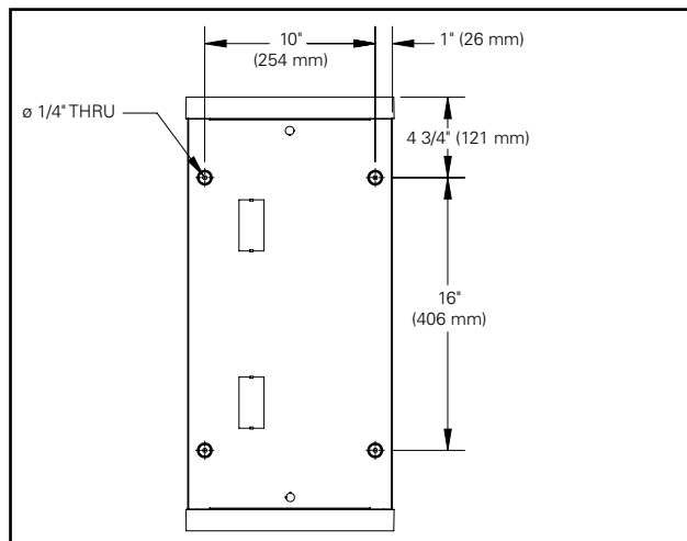
Diagrama 3: Montaje en suspensión
