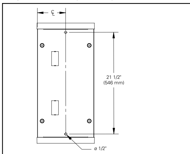
Diagrama 3: Montaje en suspensión
