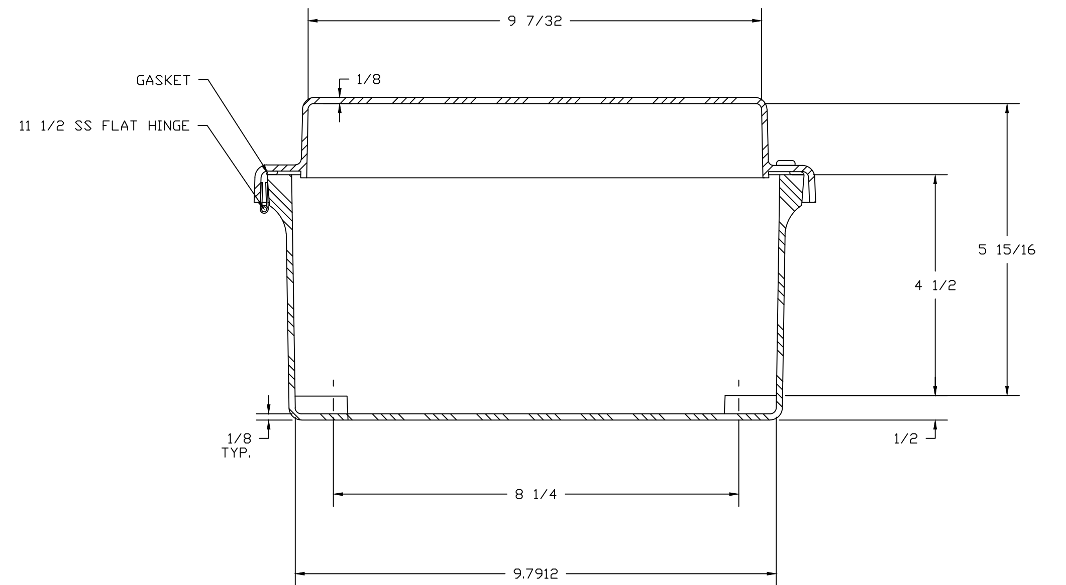
SECTION A-A
