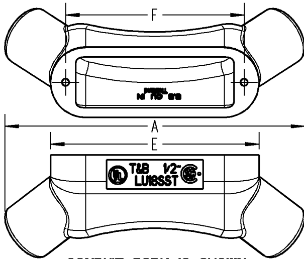
CONDUIT BODY IS SHOWN
