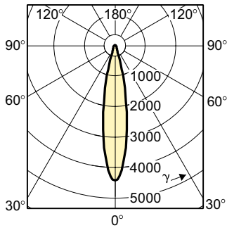
Halogen Reflector 35W GU5.3 12V 24D
