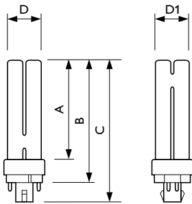
PL-C ALTO 13W/835/4P
