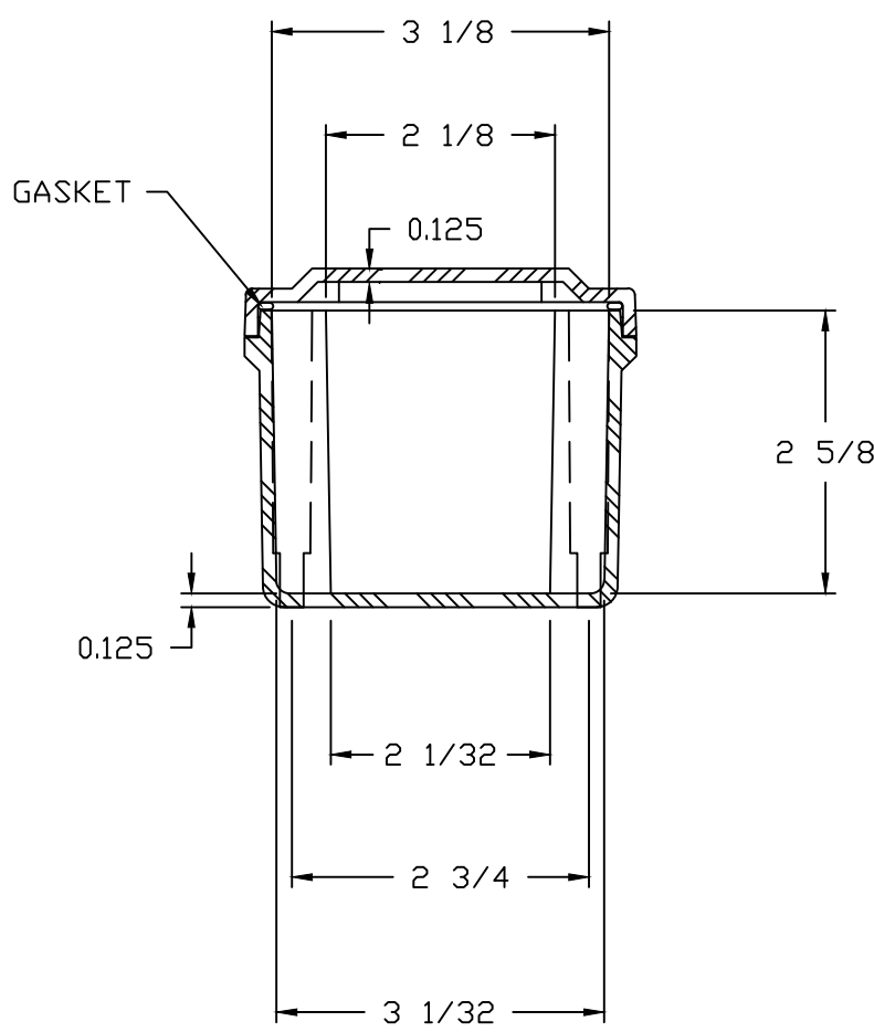
SECTION A-A
