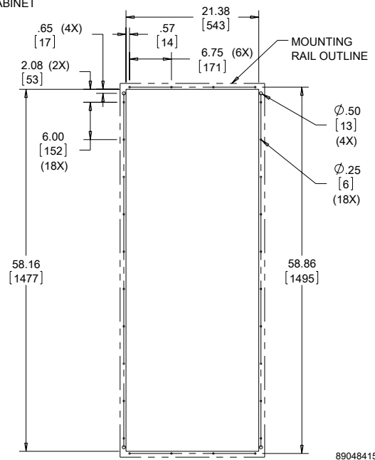
Cutout Dimensions
