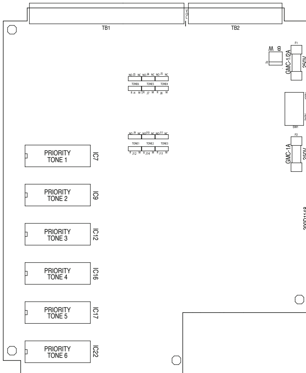
Figura 11 Placa base del 300MB
