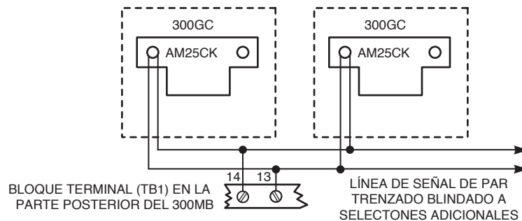
Figura 3 Conexiones del AM25CK (línea balanceada)
