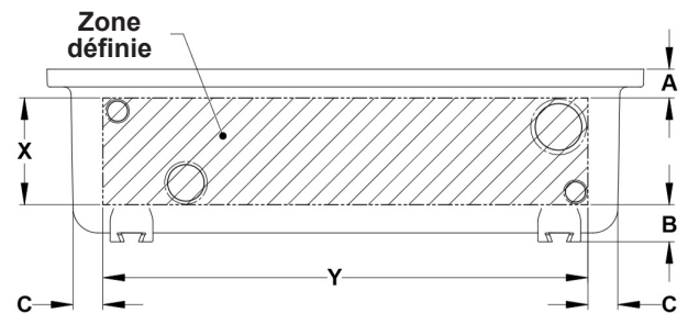
Côtés (côté long)
