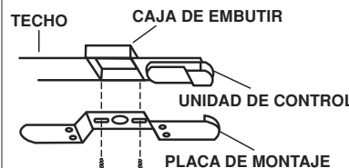
FIGURA - 5 SÓLO VENTILADORES DE MONTAJE AL TECHO
