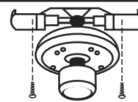
FIGURA - 4 SÓLO VENTILADORES CON VARILLA VERTICAL
