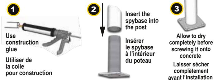
SPYBASE 22 2 X 2" OUTSIDE EXTÉRIEUR FOR SQUARE POST POUR POTEAU CARRÉ
