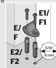
for concrete floors para pisos de concreto
