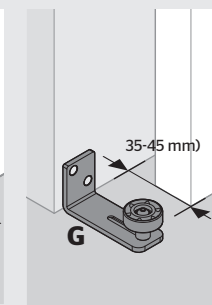
wall guide guía de pared
