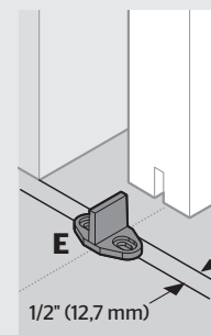
single floor guide guía de piso simple
