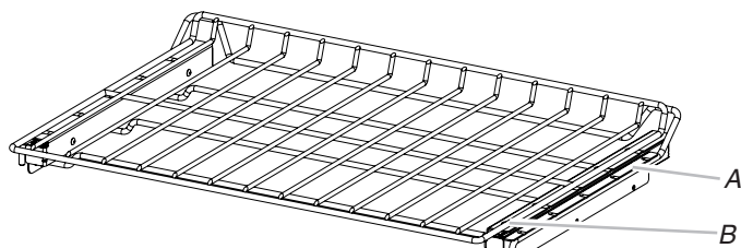
A. Glissières coulissantes B. Tablette coulissante
