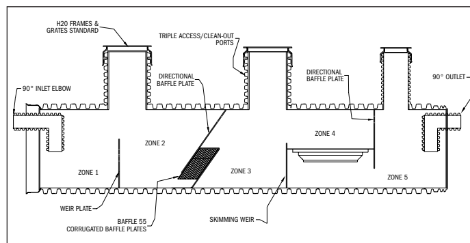
MODULE II
