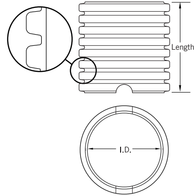
METER PITS
