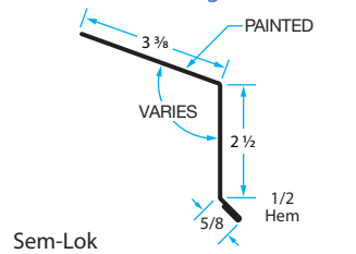
EF-5 Eave Flashing
