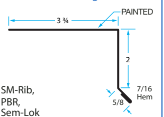
EF-3 Eave Flashing
