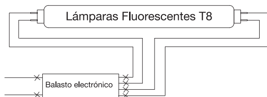
Tipo de Lastre Electrónico
