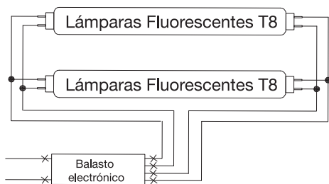
Tipo de Lastre Electrónico con Cuatro Lámparas
