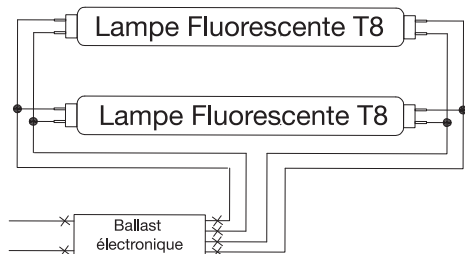
Type de ballast électronique
