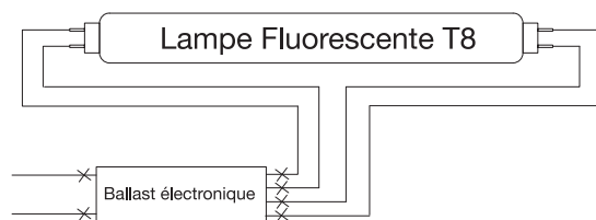
Type de ballast électronique
