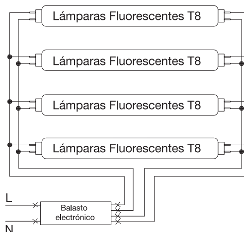
Tipo de Lastre Electrónico con Cuatro Lámparas
