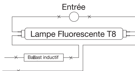
Type de ballast inductif
