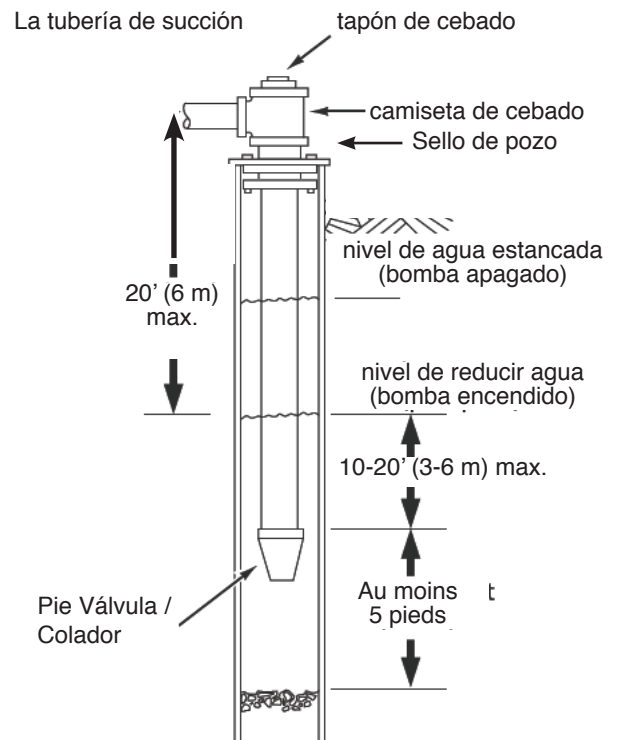
Figura 1 - Instalación de pozo entubado / cavado
