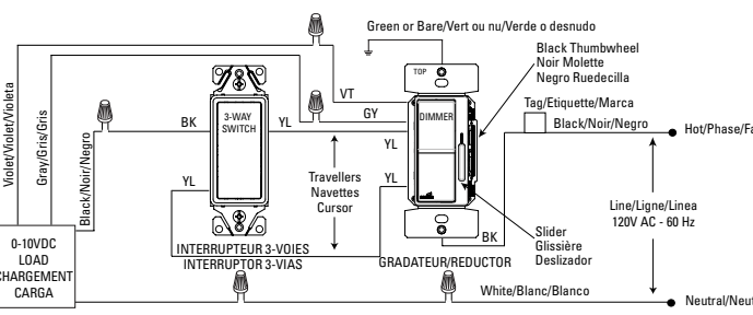
FIGURA 2: DIAGRAMA DE CABLEADO DE 3-VIAS
