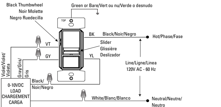
FIGURA 1: DIAGRAMA DE CABLEADO UNIPOLAR
