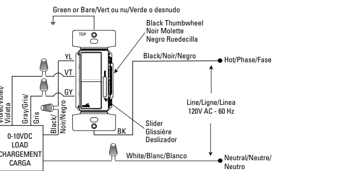
FIGURA 1: DIAGRAMA DE CABLEADO UNIPOLAR
