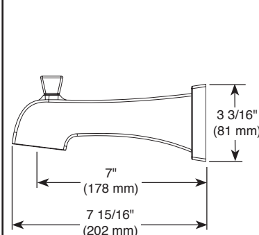
RP77901▲ (Pull-Up Diverter)
