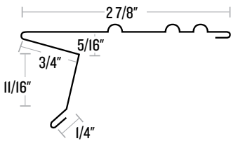
F5 OPEN DRIP EDGE
