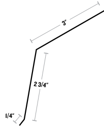
APRON FLASHING
