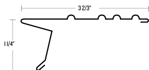
F5 1/2 DRIP EDGE
