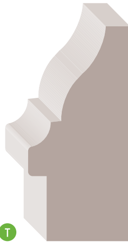
08202 1-1/16" x 2-1/4"
